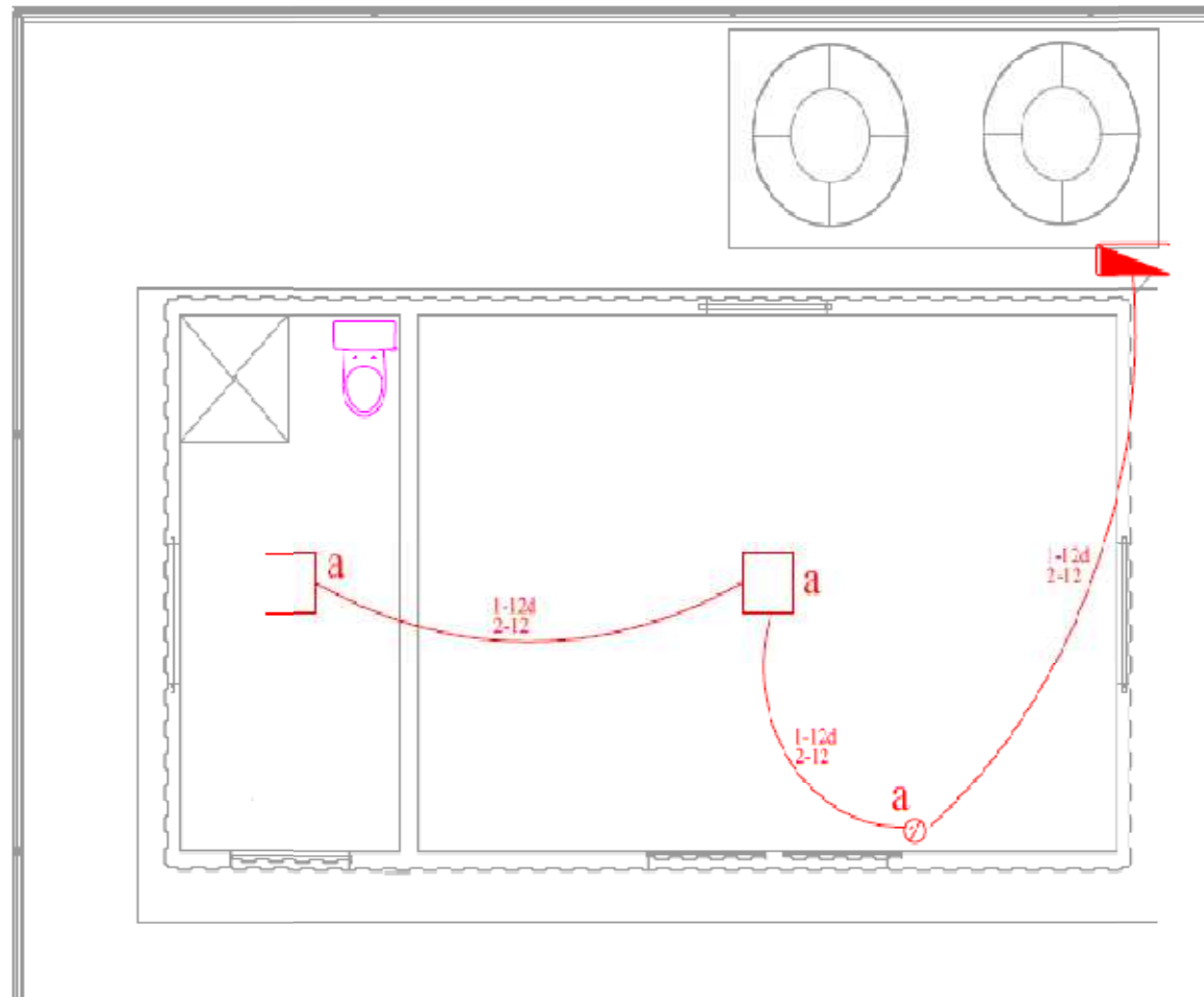
PLANTA DE INSTALACIÓN ELECTRICA LUMINARIAS
